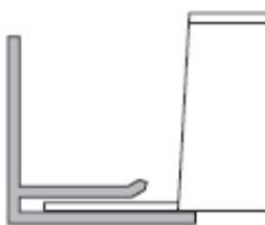
Bild 46 Alu-L-Winkel „F“ 25/25/1,5 mm
