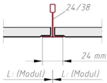
Detailschnitt
