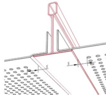
Kantenausbildung
