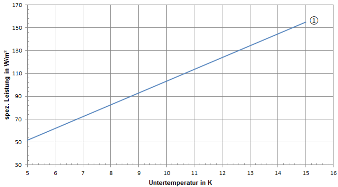
spezifische Kühlleistung
