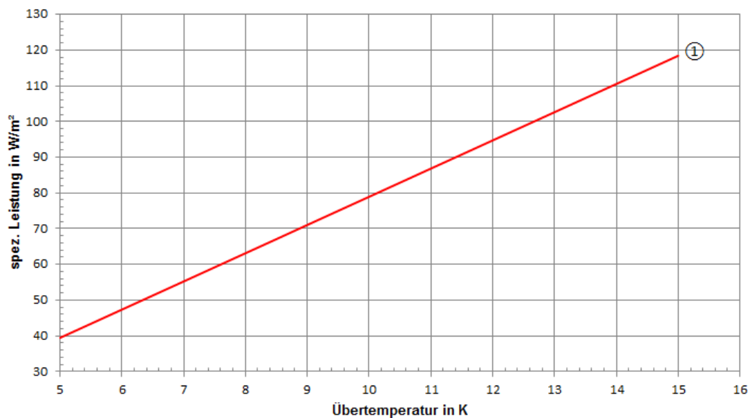
spezifische Heizleistung
